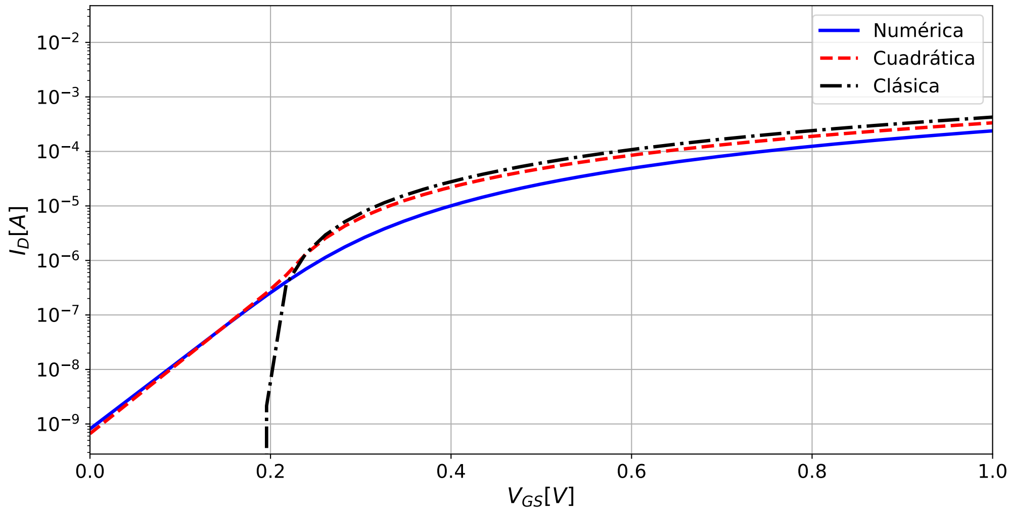
Curva de transferencia para V_{DS} = 0,5 \cdot V_{DD} = 3.25 \text{ V}
